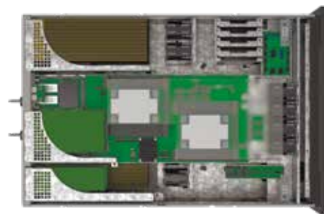
Внутреннее устройство сервера Kraftway TS3020
