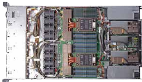
Сервер Kraftway TS5315 (внутреннее устройство)
